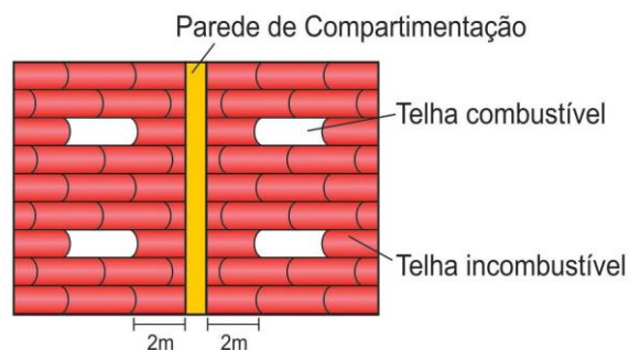
Figura 1 – Afastamento de telhas combustíveis
