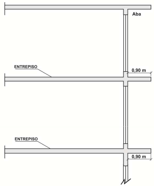
Figura A3 - Modelo de compartimentação vertical (abas)
