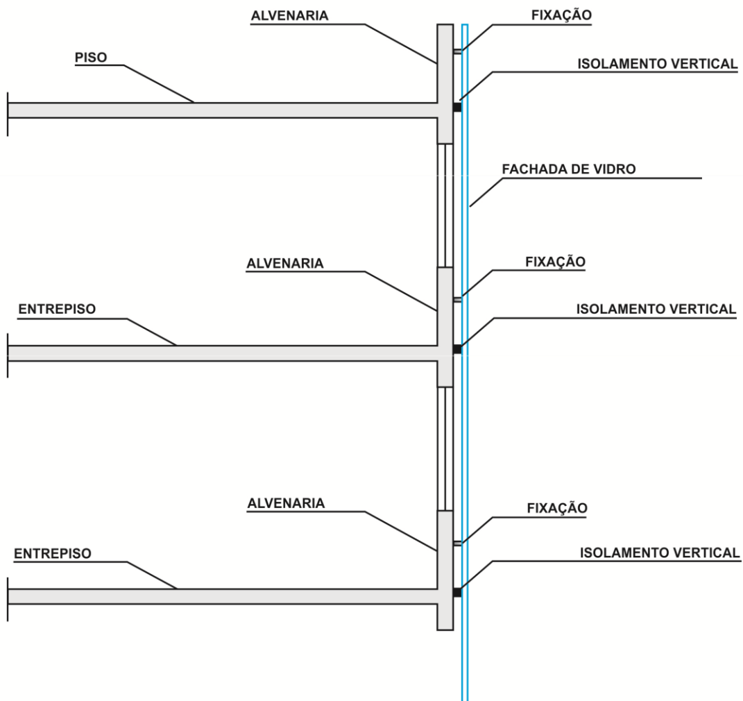
Figura A5 – Modelo de compartimentação vertical (composição entre aba e verga-peitoril)
